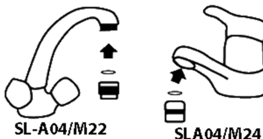
SL-A04/M22 s vnitřním závitem SLA04/M24 s venkovním závitem
